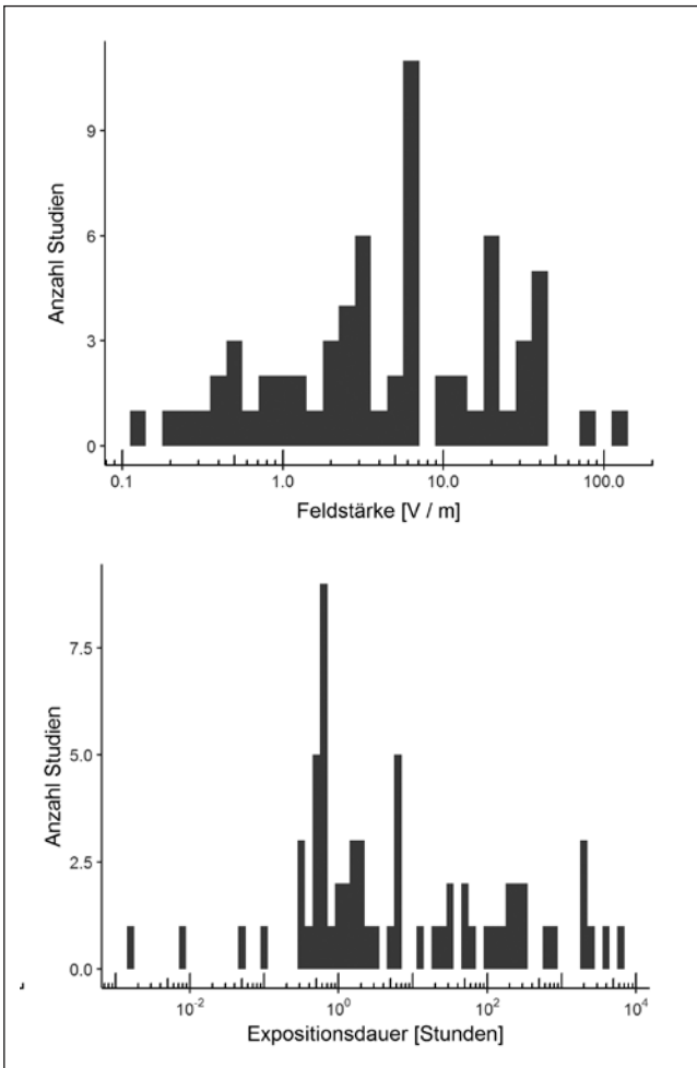
Abb. 9: Anzahl der Veröffentlichungen nach Feldstärke und Expositionsdauer (Datenpunkte aus 55 HF-EMF Studien).
