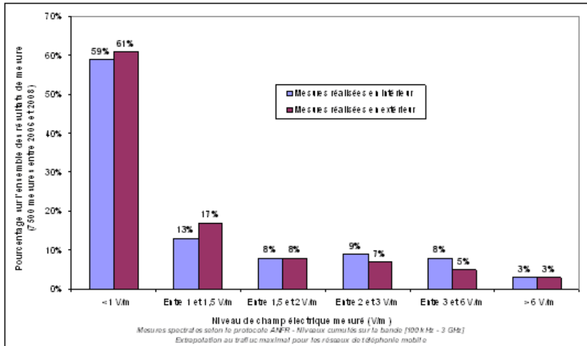
Figure 17 : distribution des résultats de mesures selon le protocole ANFR réalisées entre 2006 et 2008 (source ANFR)
