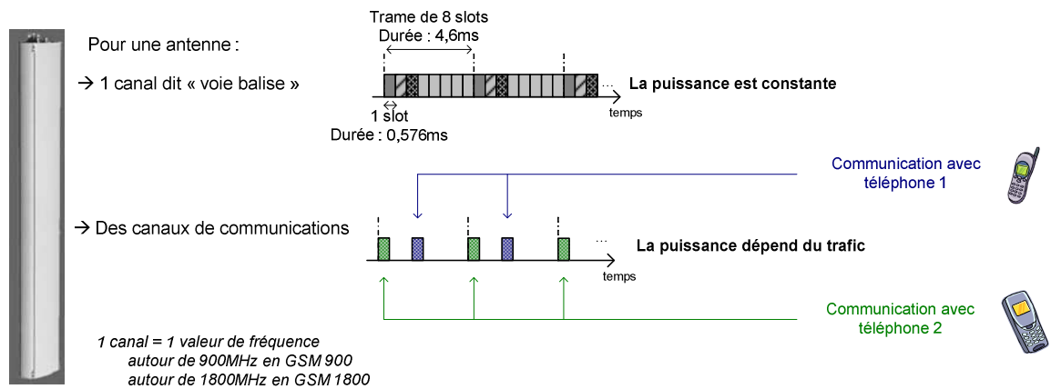
Figure 8 : canaux et voie balise en téléphonie mobile GSM
