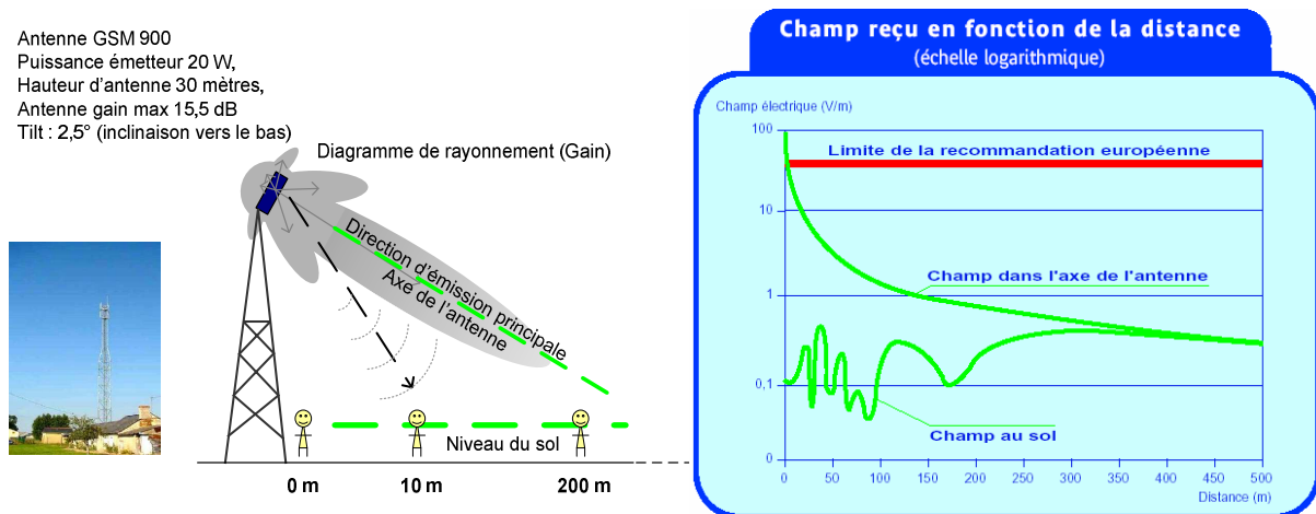
Figure 18 : exemple de mesure de champ électrique autour d'un pylône de station de base de téléphonie mobile (source ANFR)
