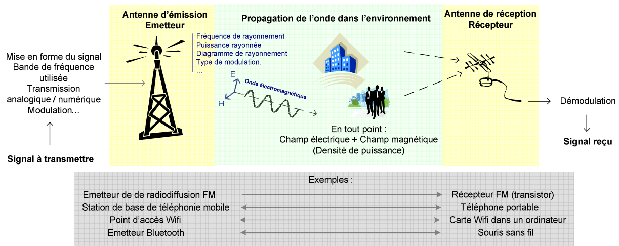
Figure 3 : principe d'une transmission radioélectrique
