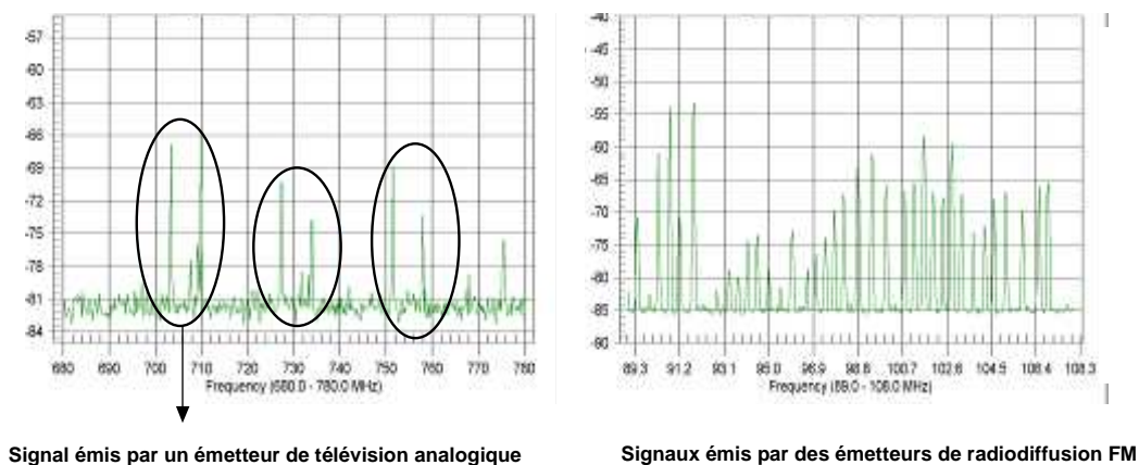
Figure 5 : exemple de spectre mesuré de radiodiffusion FM et de télévision analogique
