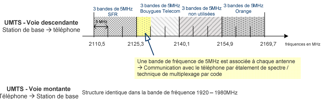
Figure 9 : bandes de fréquences de la téléphonie mobile UMTS
