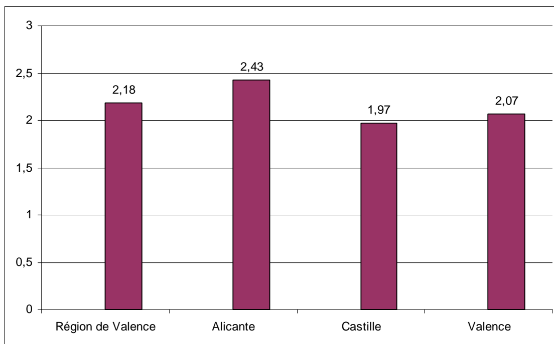
Figure 25 : Moyenne des mesures obtenues dans la région de Valence, Espagne (en V/m)
