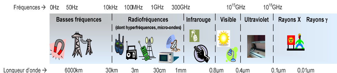
Figure 1 : spectre du rayonnement électromagnétique
