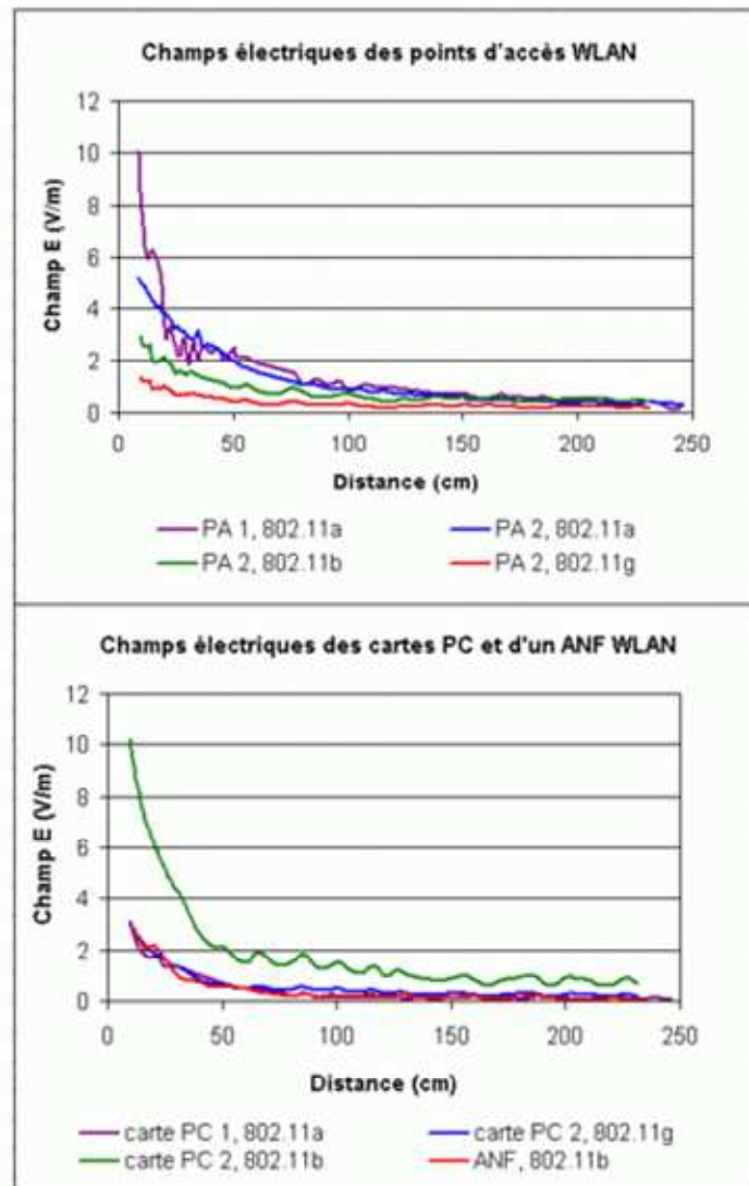
Figure 20 : niveau de champ électrique mesuré à proximité d'émetteurs Wi-Fi – Source : [Kühn, 2006]
