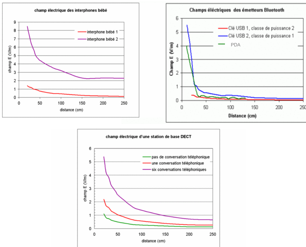
Figure 19 : niveau de champ électrique mesuré à proximité d'émetteurs radiofréquences – source : [Kramer, 2005] et [Kühn, 2006]
