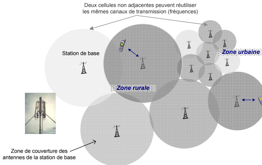
Figure 6 : réseau cellulaire de téléphonie mobile
